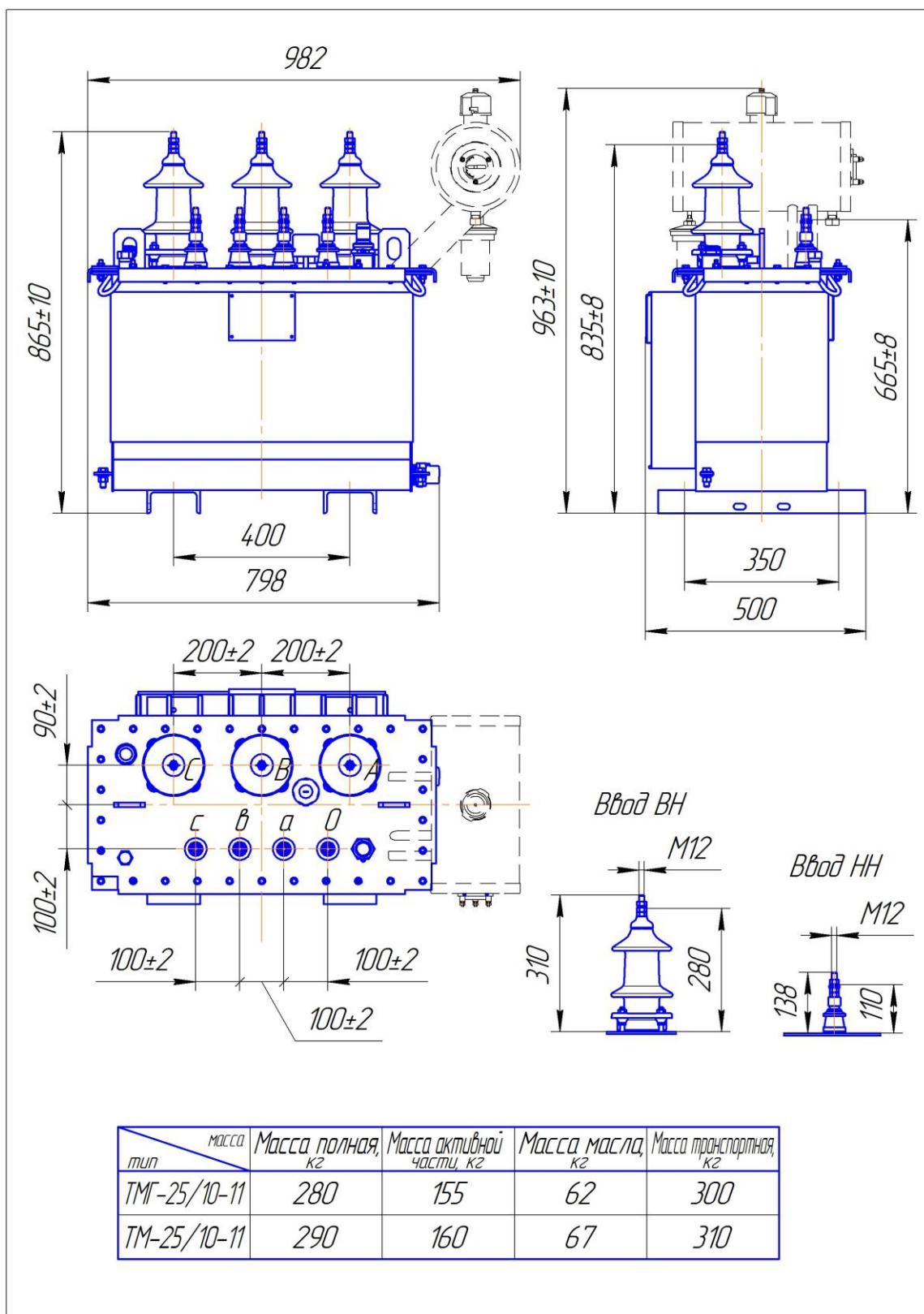
Рис. 1.1 Габаритные, установочные и присоединительные размеры трансформатора ТМГ(ТМ) - 25/10-11
