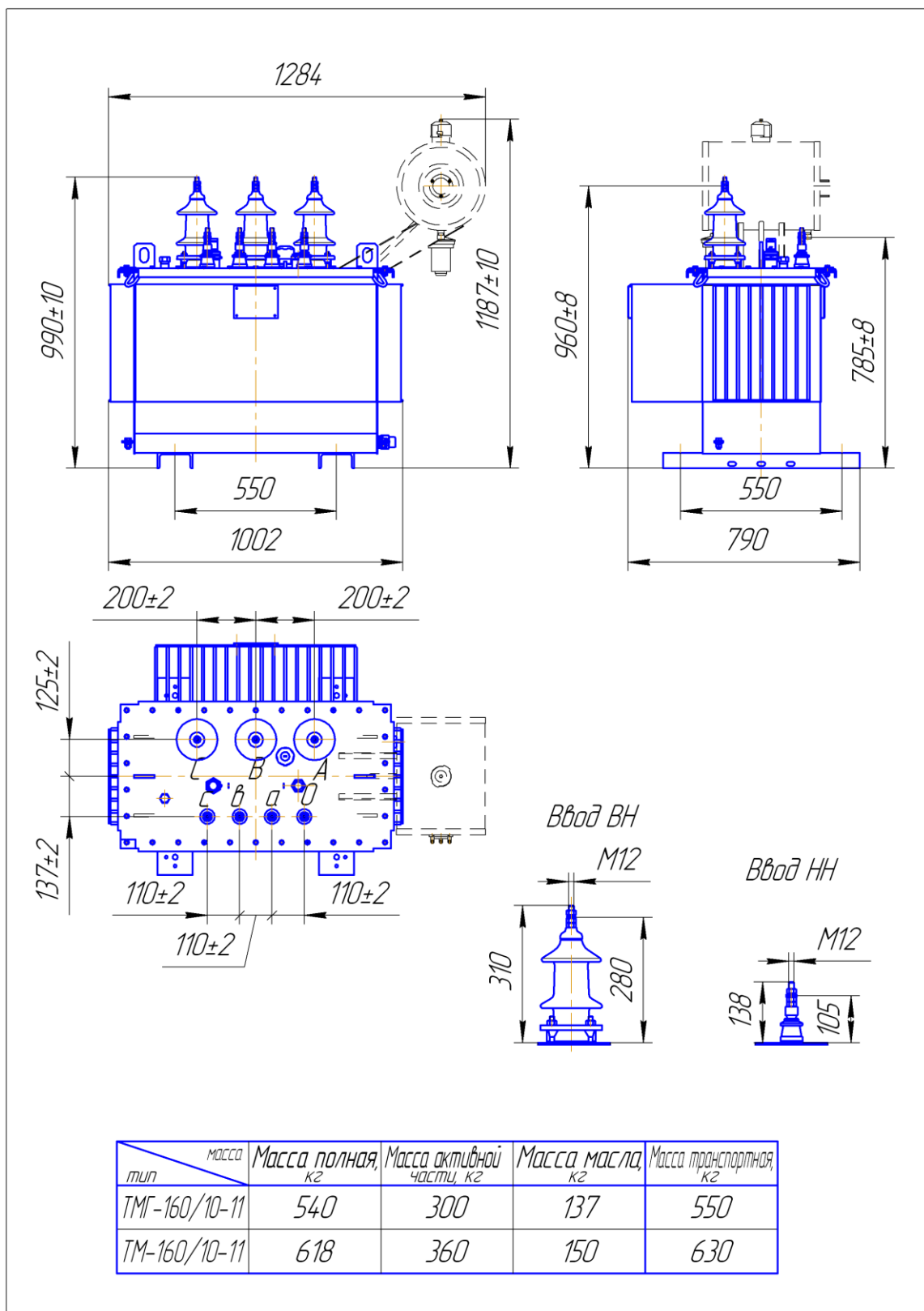
Рис. 1.5 Габаритные, установочные и присоединительные размеры трансформатора ТМ(Г) - 160/10-11
