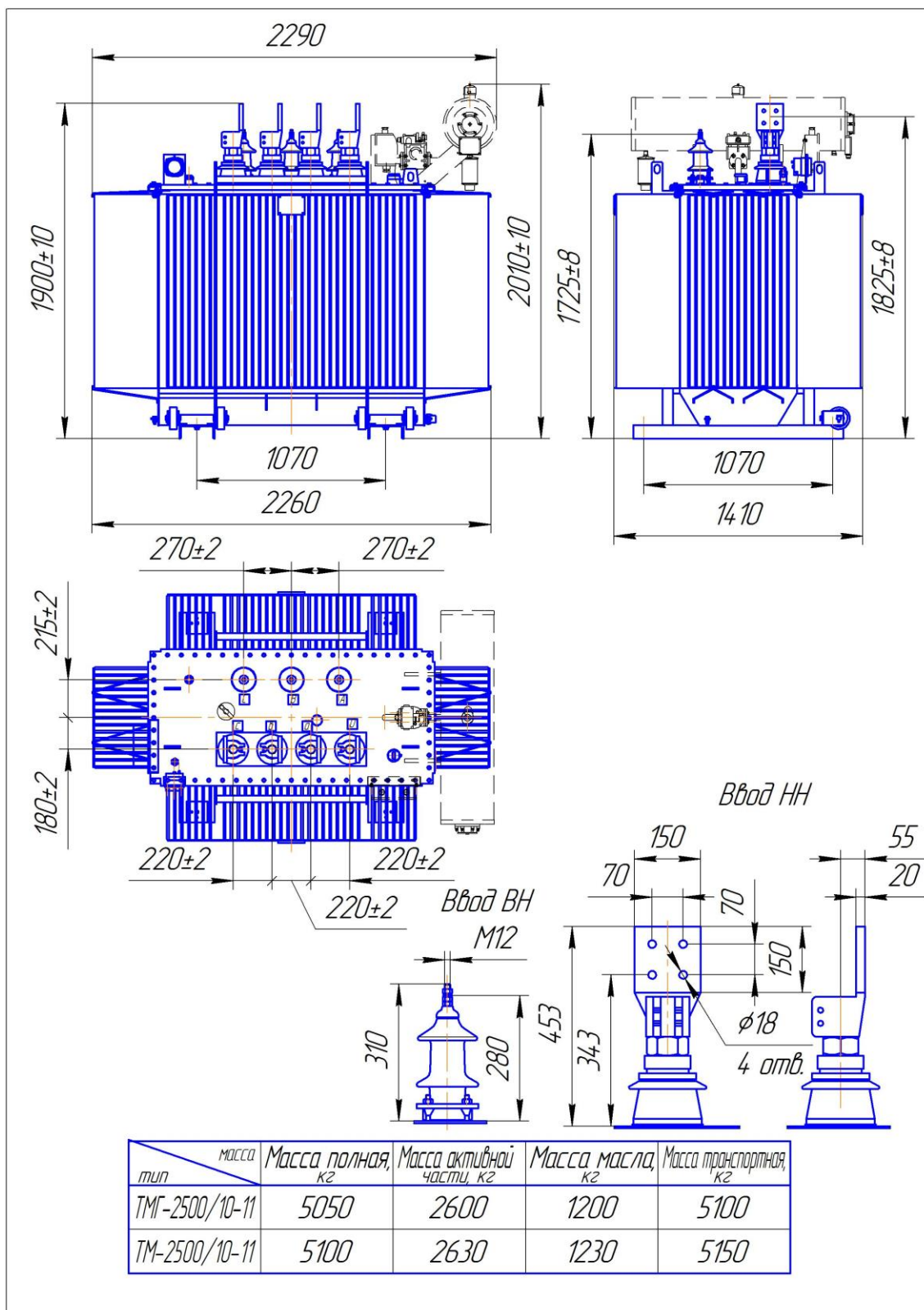
Рис. 1.19 Габаритные, установочные и присоединительные размеры трансформатора ТМ(Г) - 2500/10-11
